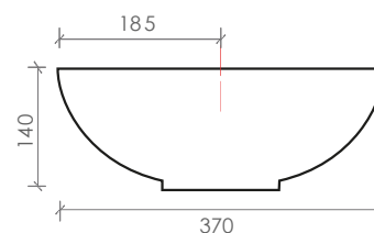
Alzado Lateral
